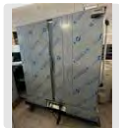
ARMARIO CALIENTA PLATOS BQ2 ARISCO
