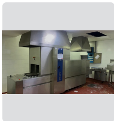
LAVAVAJILLAS TREN DE LAVADO FTNI-E-A HOBERT
