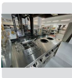
CONJUNTO COCINA ELÉCTRICA CAMPANA + SISTEMA EXTINCIÓN SILKO
