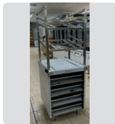
MUEBLE CON ESTANTERIA + GUIAS BANDEJERAS INOX
